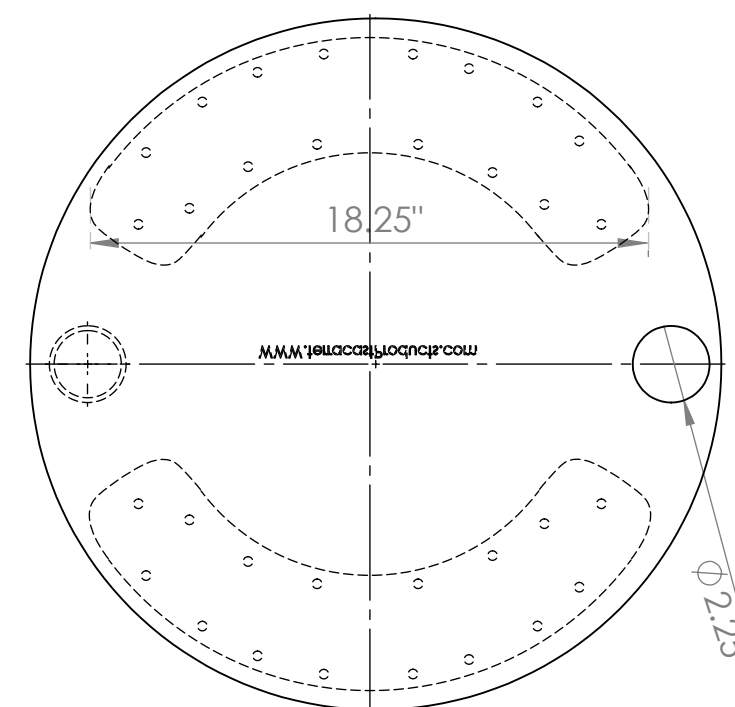
BOTTOM
